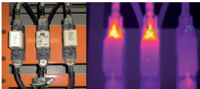
Figura 6 - Mau contato nas pinças dos fusíveis Fonte: MHF Manutenção Preditiva. Disponível em: < www.mhfpreditiva.com.br >. Acesso em: 03 jun. 2011.
