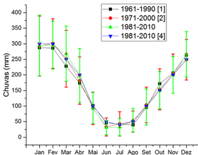
Figura 7: Normais climatológicas para 1961-1990, 1971-2000 e 1981-2010 contidas na dispersão em torno da média mensal de qualquer uma das climatologias
