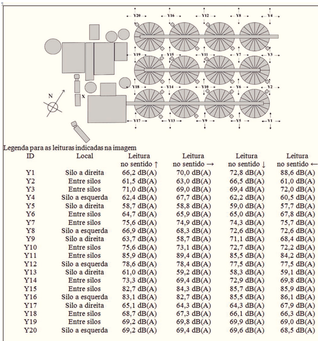
Figura 2. Indicação do ponto de instalação do Decibelímetro X e dados obtidos do Decibelímetro Y
