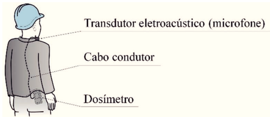
Figura 1. Detalhe da colocação do dosímetro do operador avaliado
