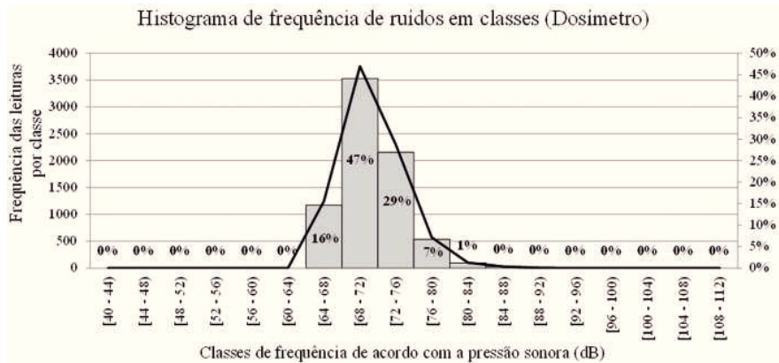
Figura 6. Distribuição de frequência das pressões sonoras segundo classes de dB(A) para o Dosímetro
