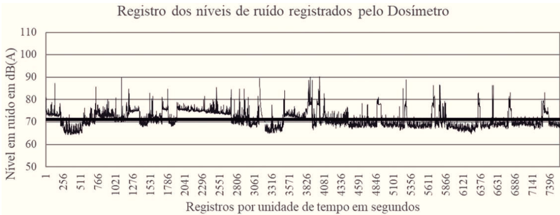
Figura 4. Comportamento do ruído ao longo do tempo registrado pelo Dosímetro
