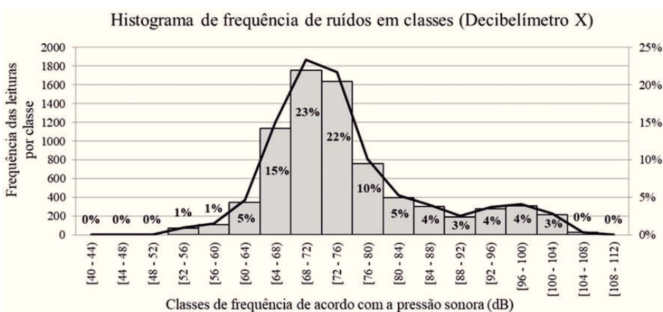
Figura 5. Distribuição de frequência das pressões sonoras segundo classes de dB(A) para o Decibelímetro X
