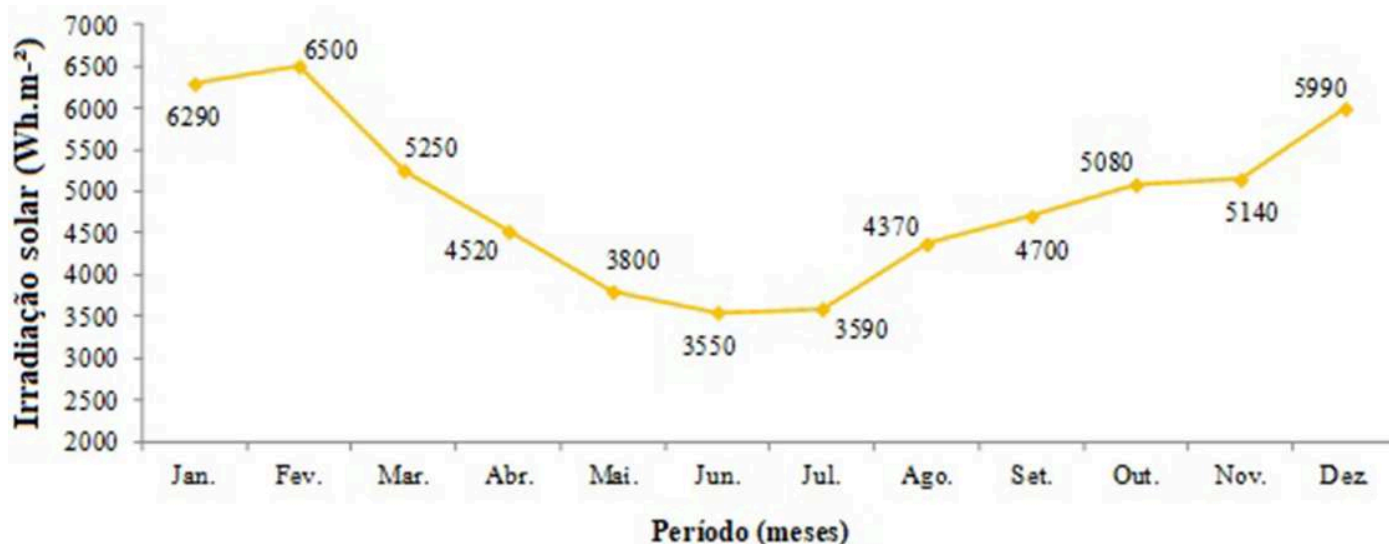
Figura 12. Gráfico de irradiação solar no plano horizontal, em \text{Wh.m}^{-2} , na latitude de 21^{\circ}44' e longitude de 41^{\circ}19'
