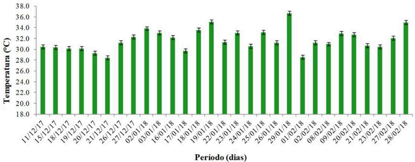
Figura 17. Gráfico de temperatura ambiente do período do experimento, em °C
