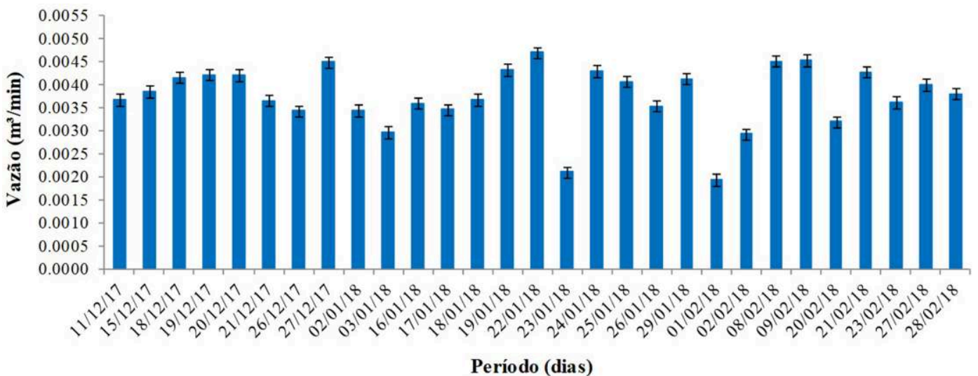
Figura 16. Gráfico de vazão diária de bombeamento, em m 3 /min
