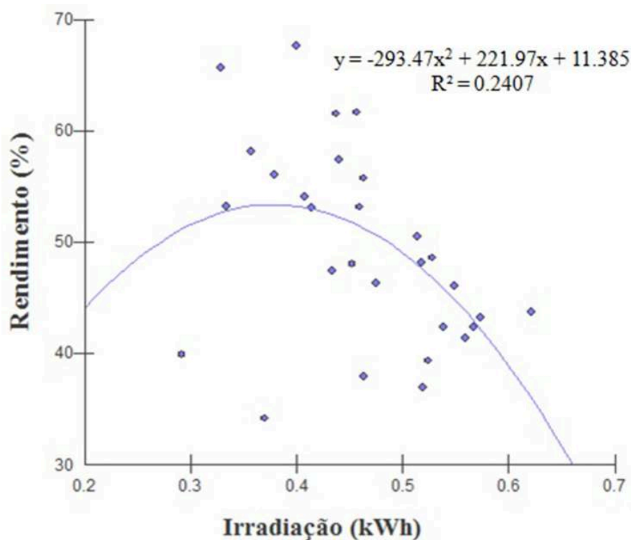
Figura 20. Diagrama de dispersão dos dados de Irradiação Solar e Rendimento
