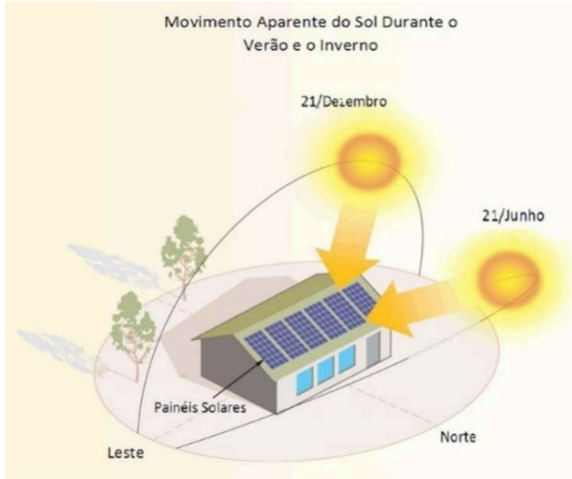
Figura 4. Movimento aparente do Sol em relação à Terra responsável pela formação dos Solstícios de inverno e verão
