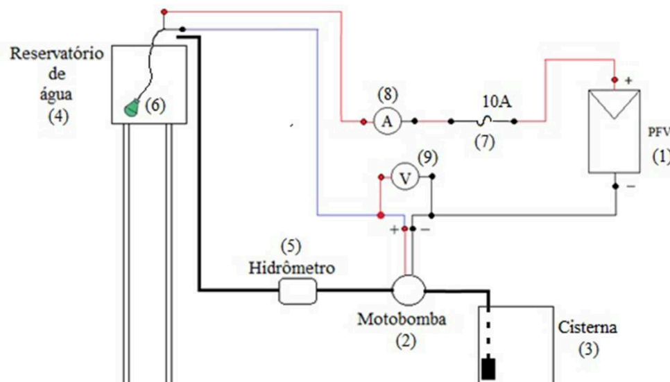
Figura 11. Montagem proposta para o sistema elétrico-hidráulico
