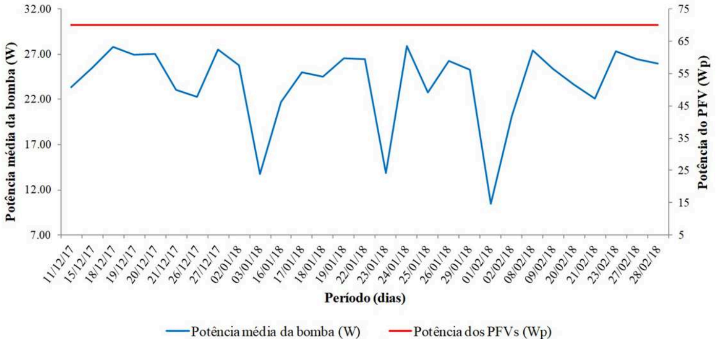
Figura 15. Gráfico de potência média diária da bomba (W) e potência nominal dos MFVs (W p )
