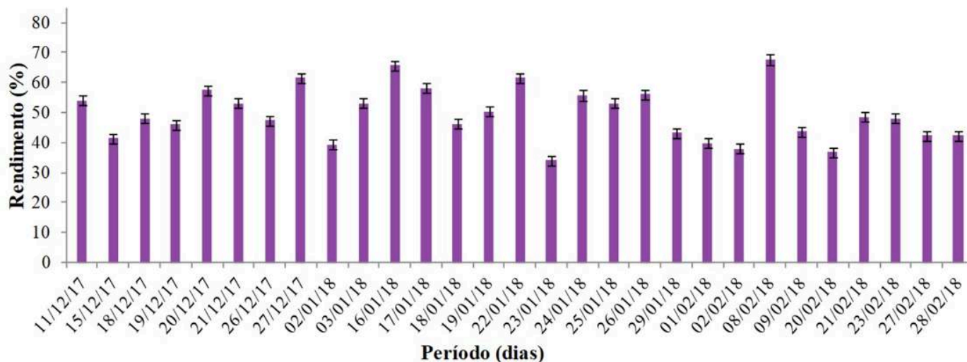
Figura 18. Gráfico de rendimento do sistema fotovoltaico de bombeamento, em %
