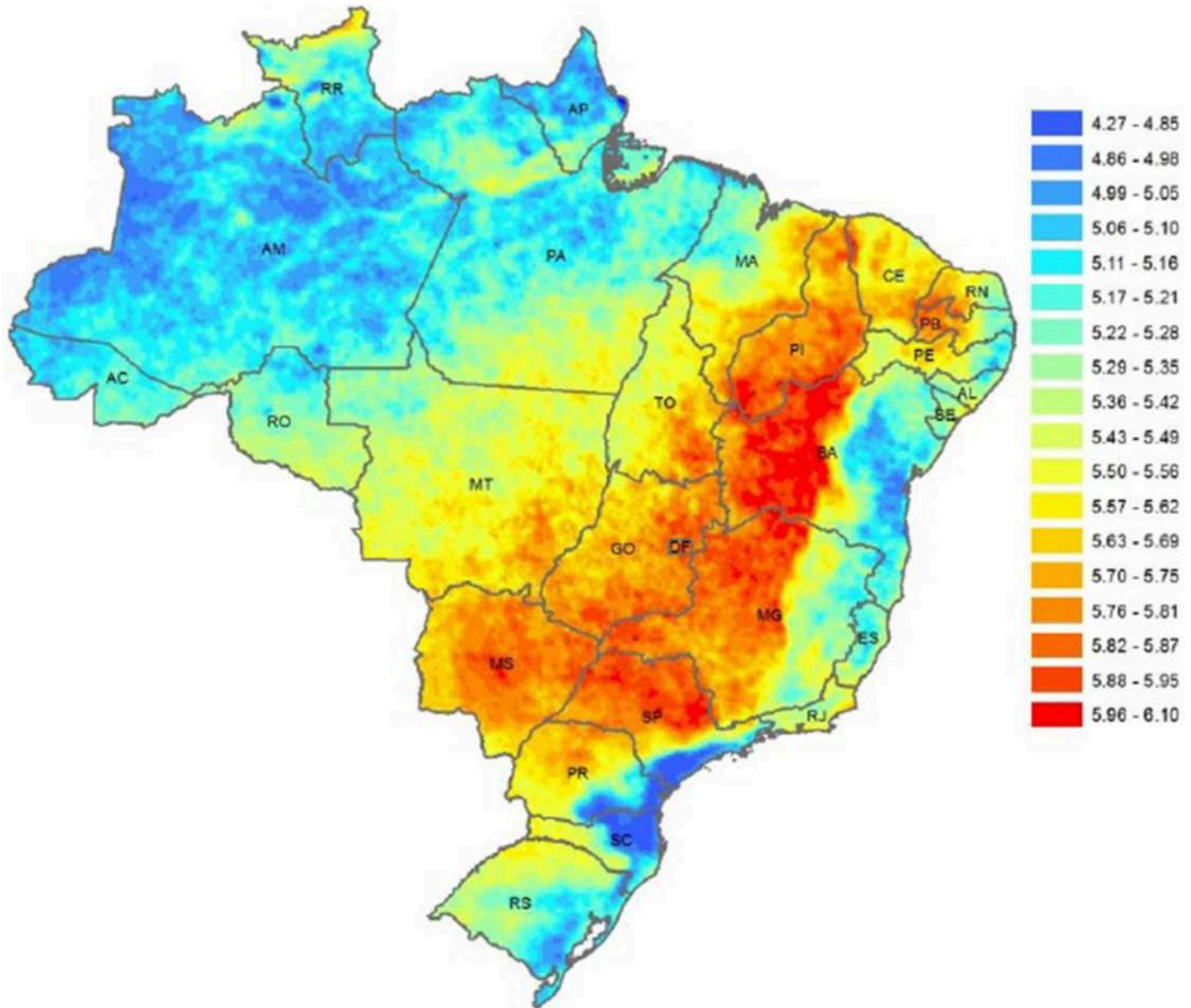
Figura 1. Irradiação total em plano (kWh.m -2 /dia)
