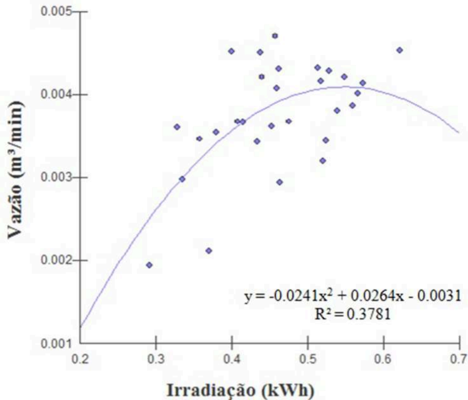
Figura 19. Diagrama de dispersão dos dados de Irradiação e Vazão coletados
