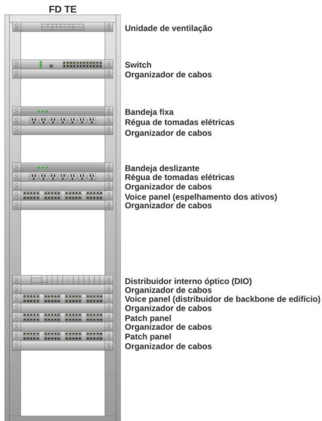
Figura 5. Plano de face do rack
