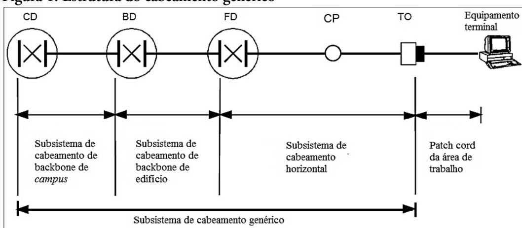
Figura 1. Estrutura do cabeamento genérico
