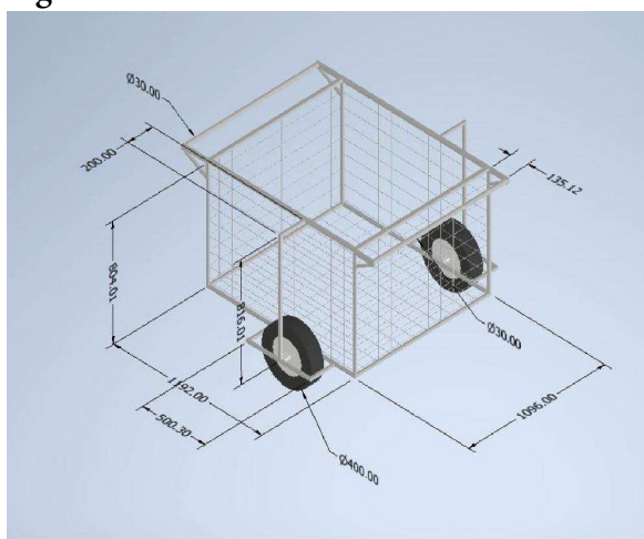
Figura 2. Modelo de carrinho com dois varais de tamanhos iguais
