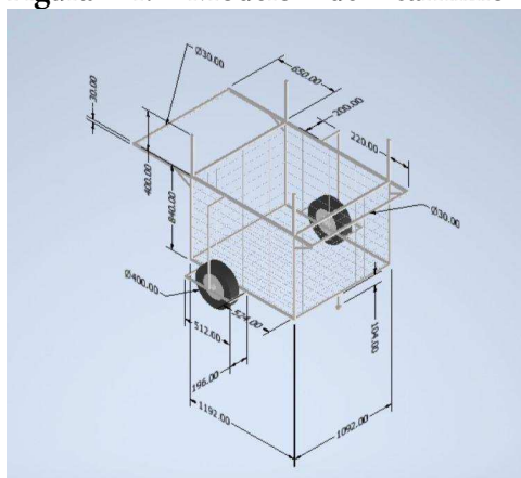
Figura 4. Modelo de carrinho após alterações sugeridas pela atividade de simulação
