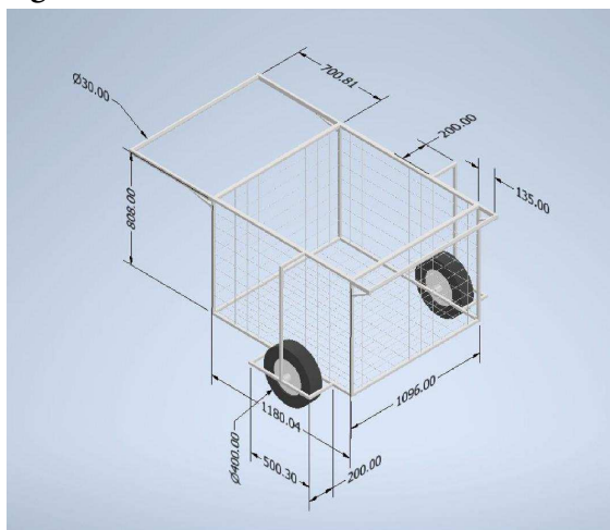
Figura 1. Modelo de carrinho com dois varais de tamanhos distintos
