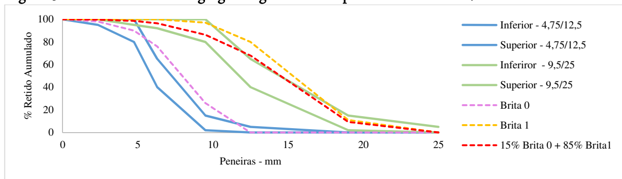
Figura 3. Granulometria de agregados graúdos comparativa com NBR 7211
