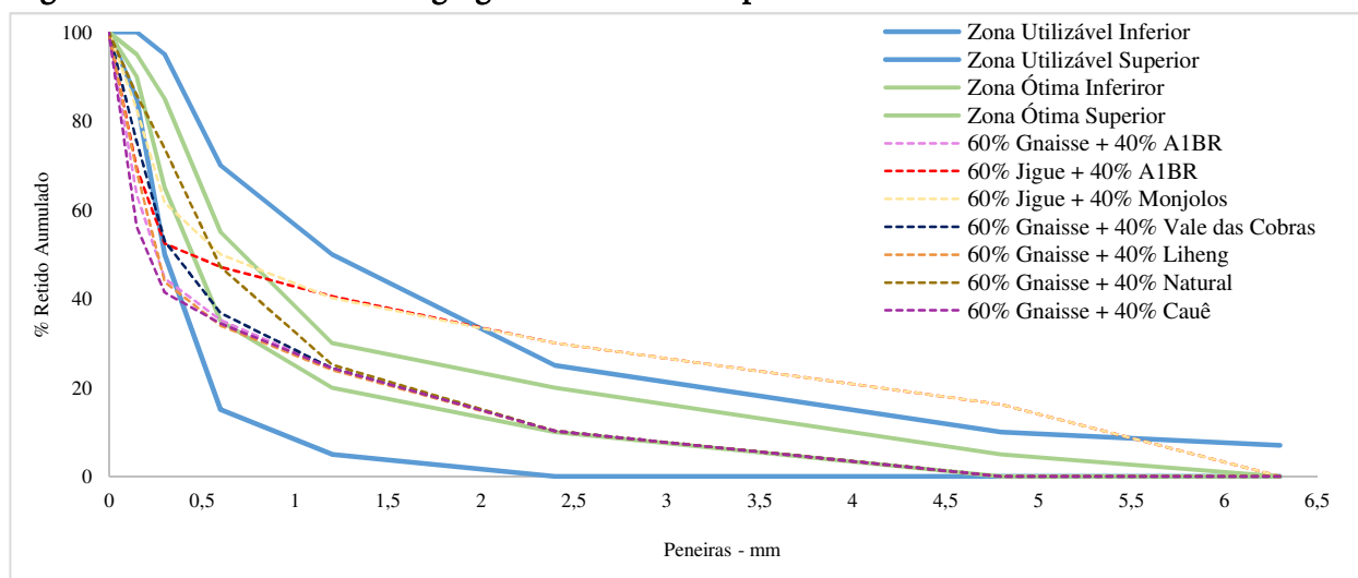
Figura 2. Granulometria de agregados miúdos comparativa com NBR 7211
