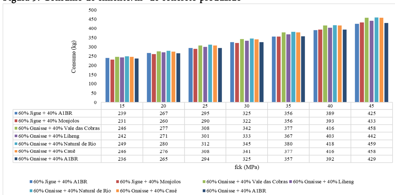
Figura 5. Consumo de cimento/m 3 de concreto produzido
