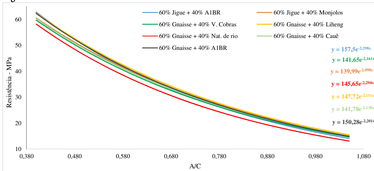
Figura 4. Curva Curvas de Abrams - 28 dias
